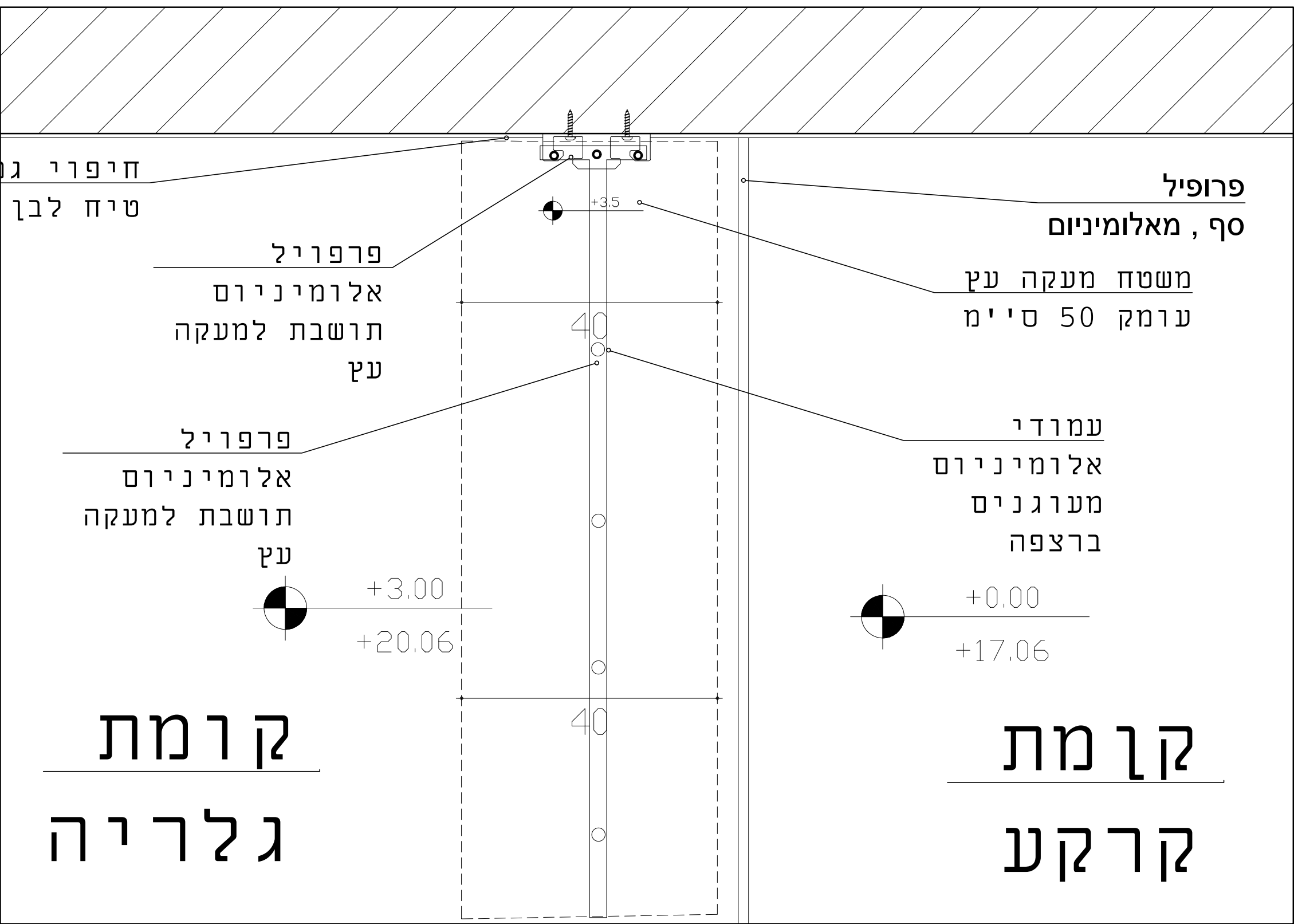
פרט-C 1:5 סף דלת הזזה יציאה למרפסת דק
