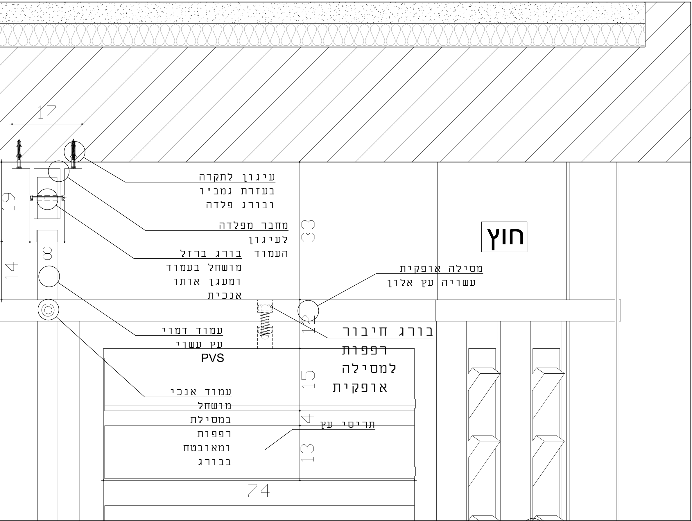
פרט-B 1:5
