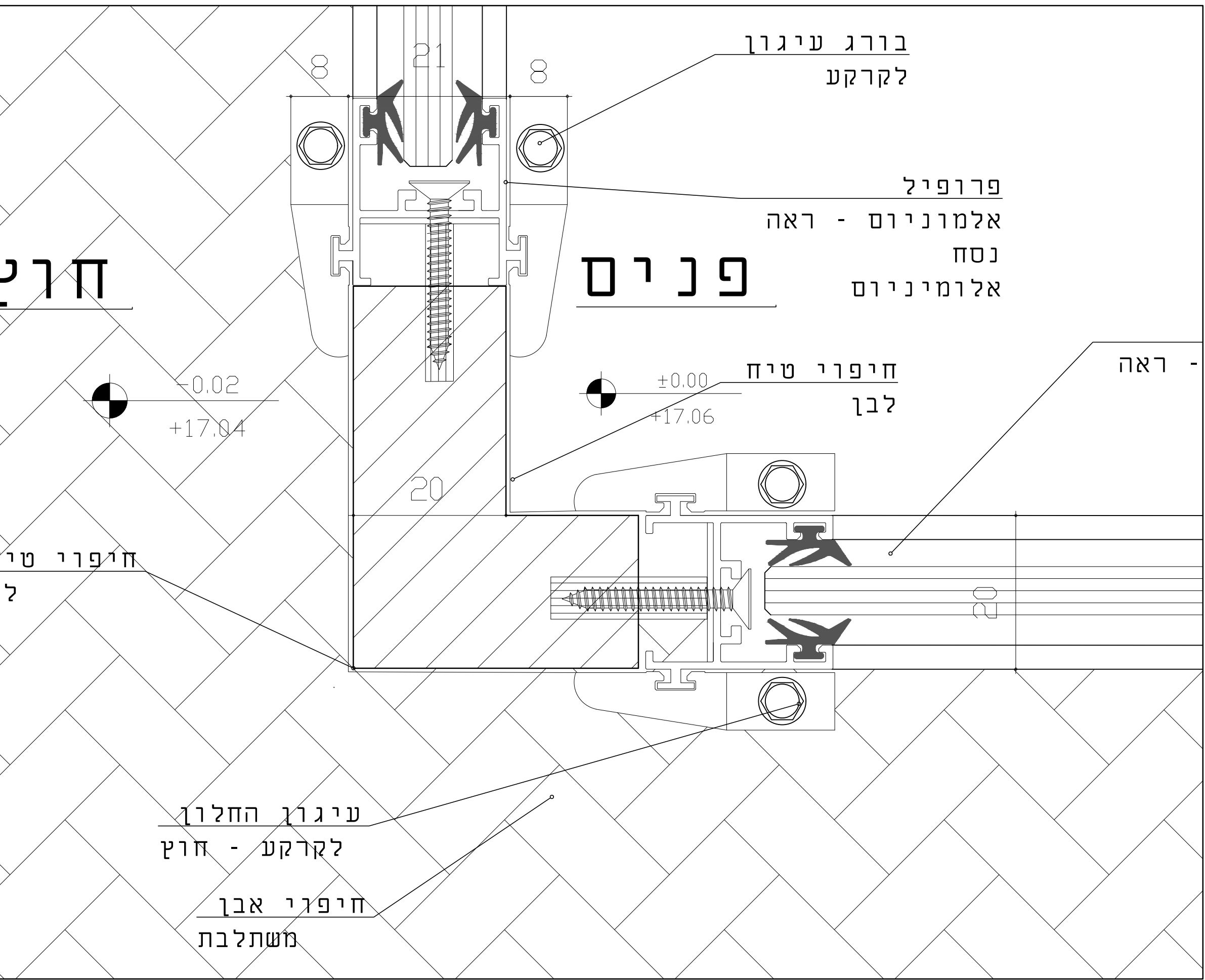
פרט-D חיבור וירטיננה לקרקע 1:5
