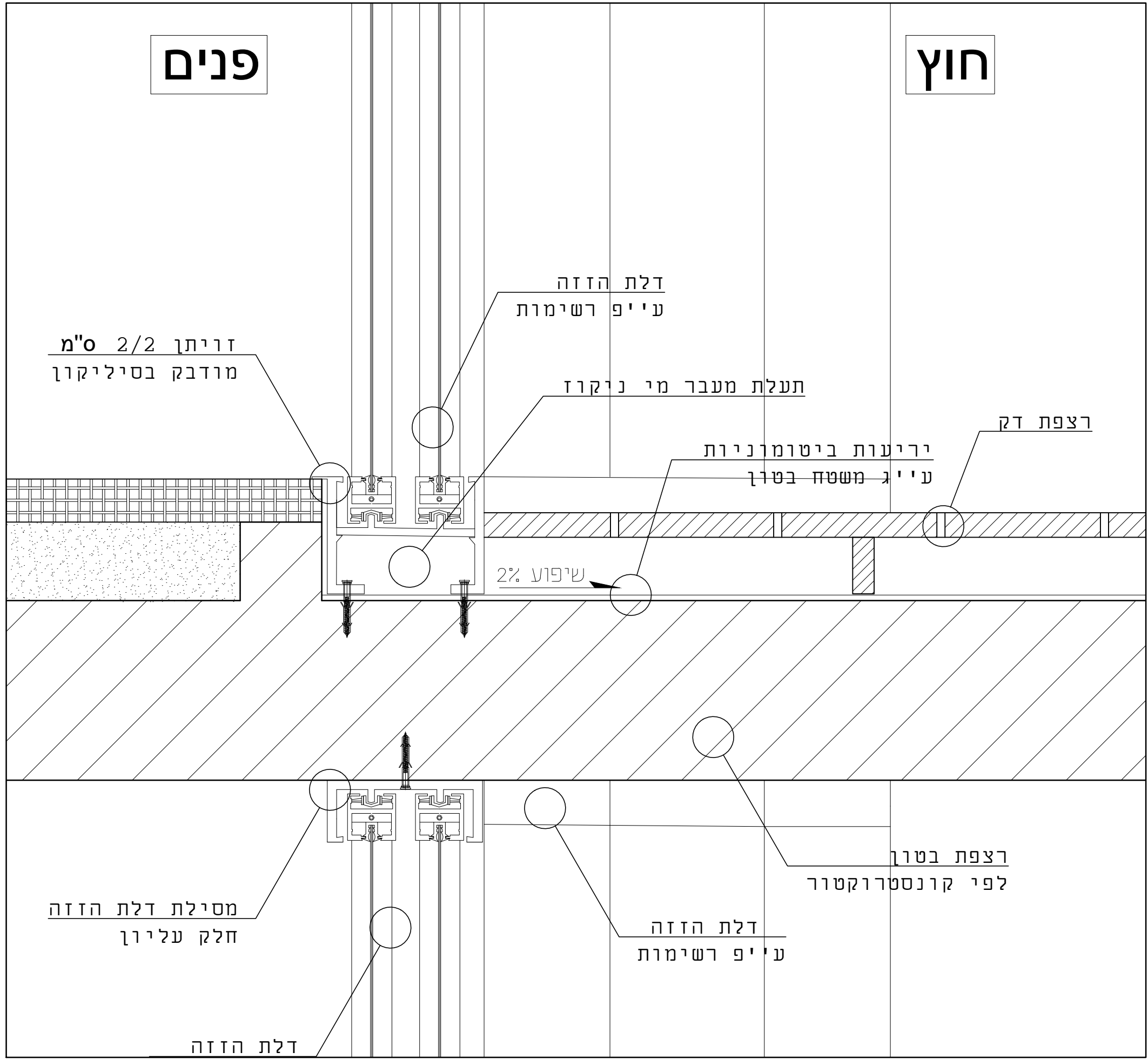
פרט-C 1:5 סף דלת הזזה יציאה למרפסת דק
